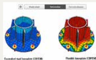
Abb. 8: Vergleich der Verformungen
