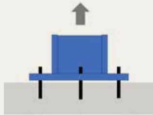
Abb. 2: Zuglast wird gleichmäßig auf alle Dübel verteilt
