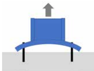
Abb. 4: Abstützkräfte in der Nähe der Kanten
