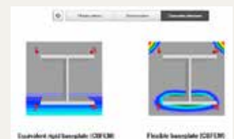
Abb. 10: Vergleich der Druckzone
