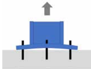
Abb. 5: Umverteilung der Lasten in der Dübelgruppe
